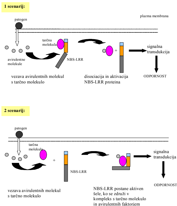
Slika 1: Scenarija, ki ponazarjata delovanje R proteinov pri hipotezi nadzovanja Figure 1: Guard hypothesis scenarios for R protein function
